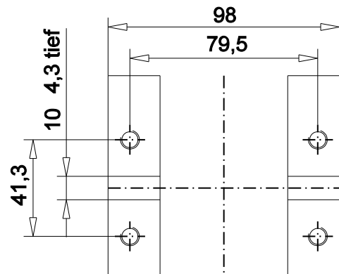
Maße - Getriebefuß
