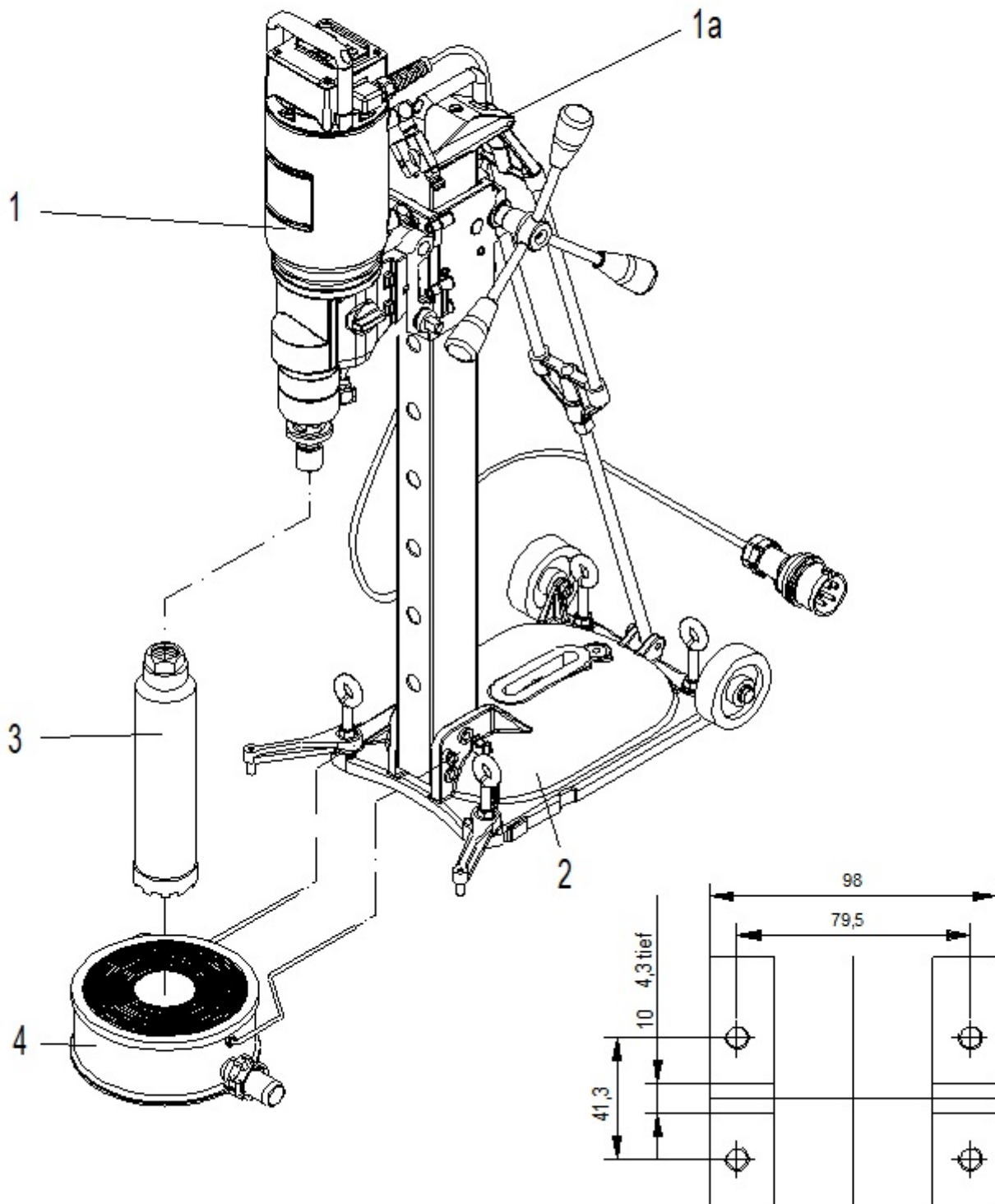
Maße - Getriebefuß
